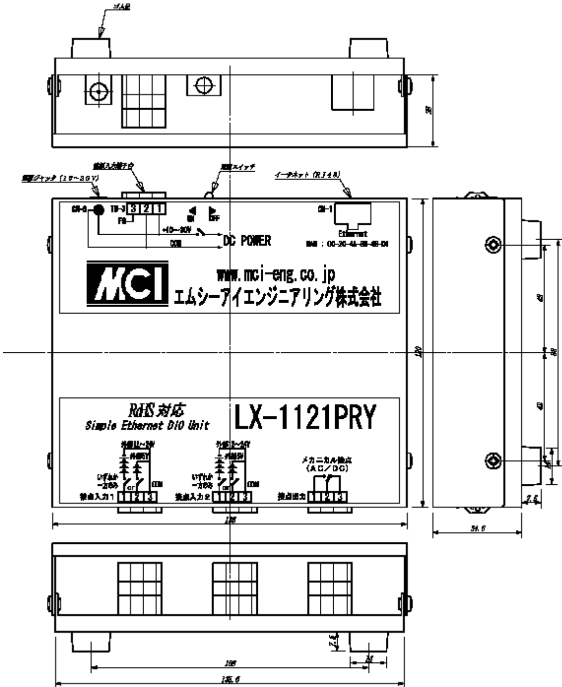
( a ) LX - 1121PRYの外観
