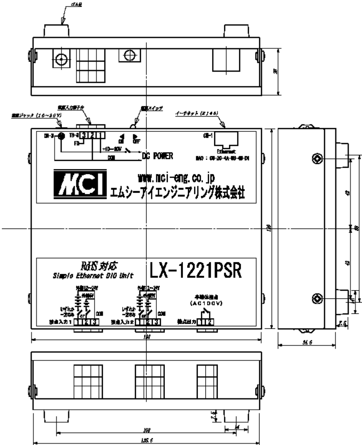
(b) LX - 1221PSRの外観
